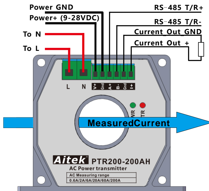
4-11 整体接线示意图
